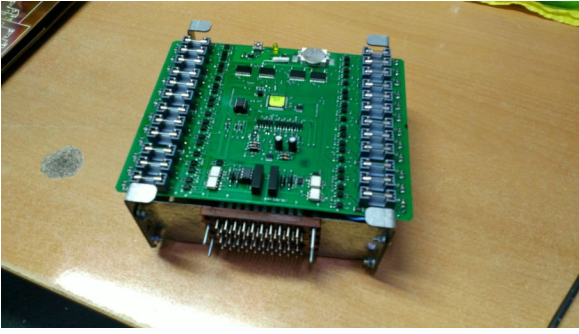
- блок электронный КДУ
